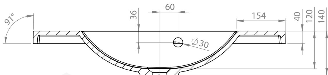
PRZEKRÓJ N-N SKALA 1:7
